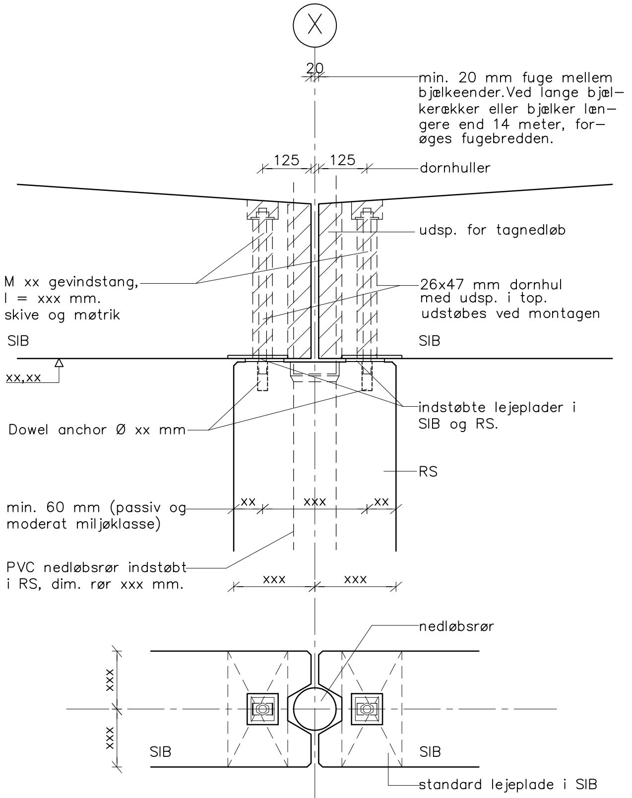
Samling mellem RS / SIB-bjælker (dornsamling – indstøbt nedløbsrør i RS)
